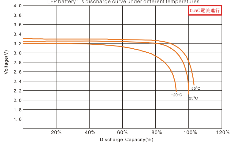
不同环境温度下 LFP类电池的放电特性曲线
