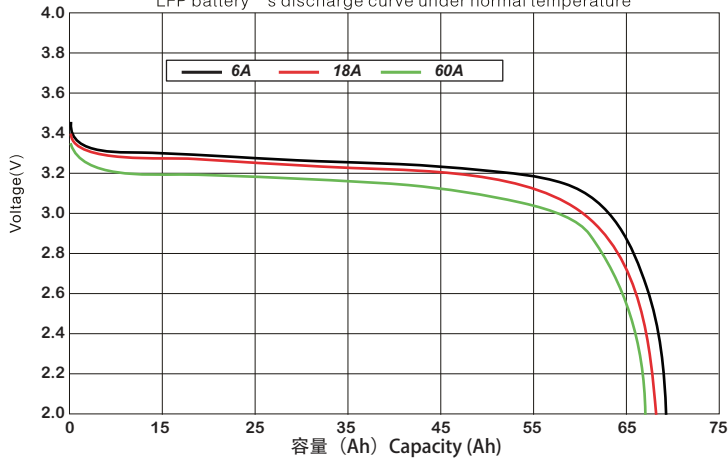
常温下LFP类电池的放电特性曲线
