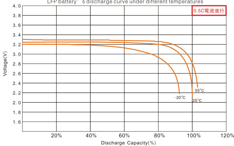
不同环境温度下 LFP类电池的放电特性曲线 LFP battery's discharge curve under different temperatures
